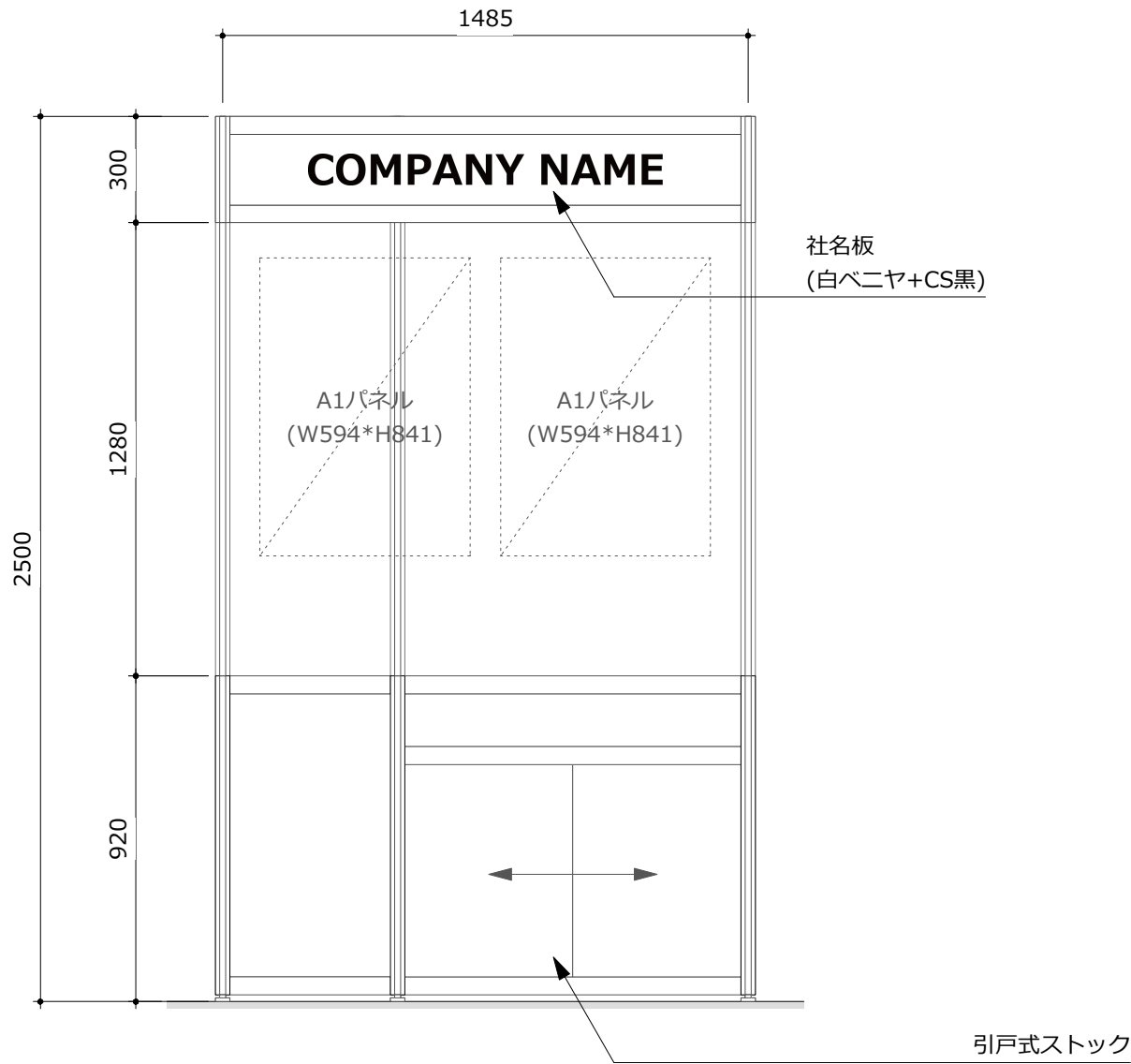
Elevation
